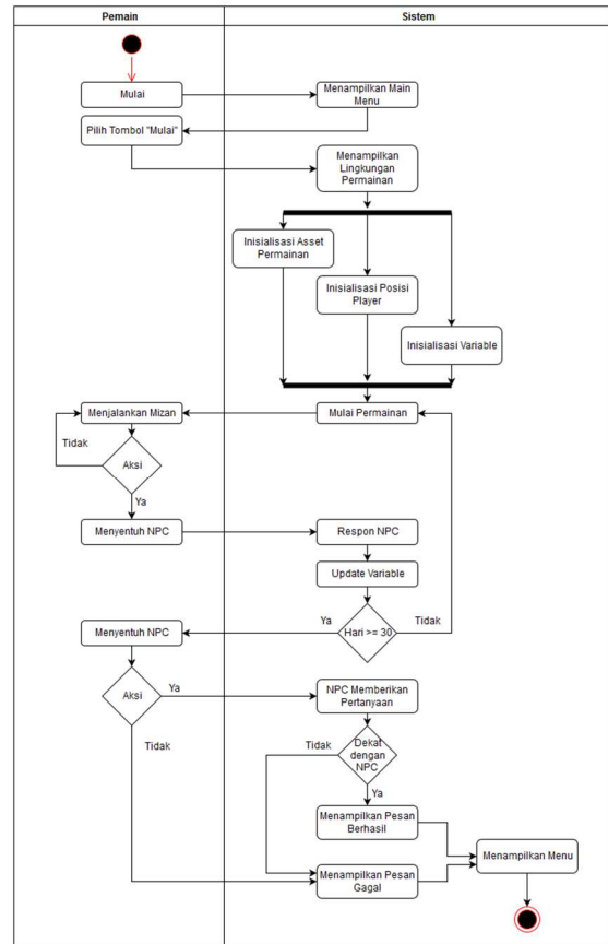
Gambar 5. Activity Diagram untuk “Play”
