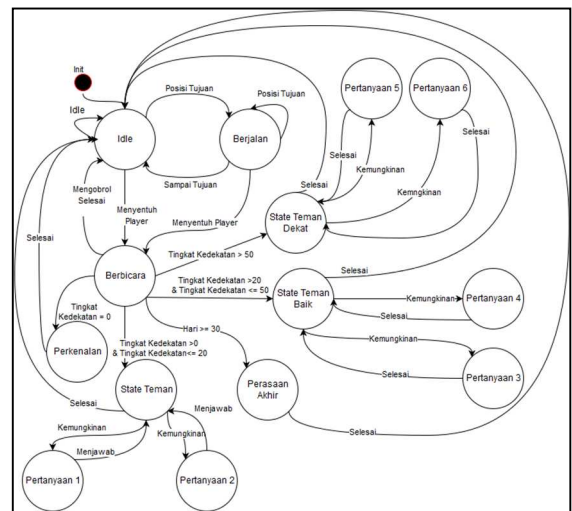
Gambar 3. State Diagram NPC Utama
